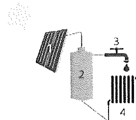
1. Zonnecollector [2] Opslagvat warm water [3] Sanitair warm water [4] Radiator voor ruimteverwarming (bij aanwezig)
