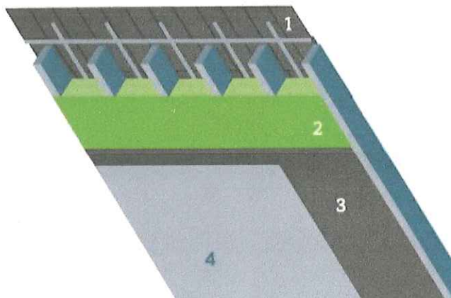
1. Onderdak | 2. Isolatie | 3. Dampschermbekleding | 4. binnenafwerking
