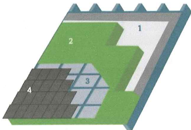
1. Dampschermbekleding | 2. Isolatie | 3. Onderdak | 4. Dakbedekking
