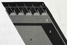
1. Onderdak | 2. Isolatie | 3. Dampscherm | 4. binnenafwerking
