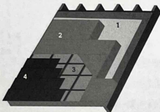
1. Dampscherm | 2. Isolatie | 3. Onderdak | 4. Dakbekleding
